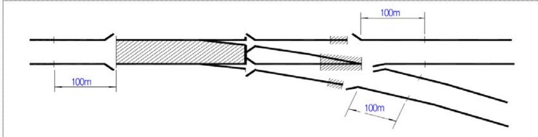
그림 3.3-2 절단한 레일 끝부분 틀어놓음
