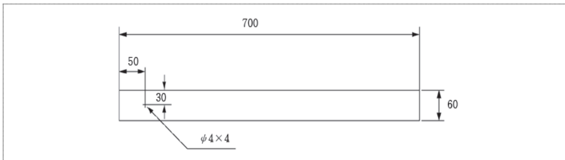
그림 3 레일 용접부 탐상용 대비 시험편(단위 mm)
