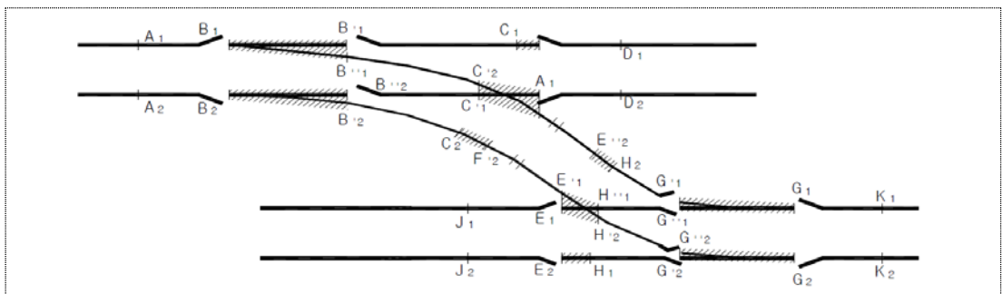
그림 3.3-4 건널선의 장대레일 재설정
