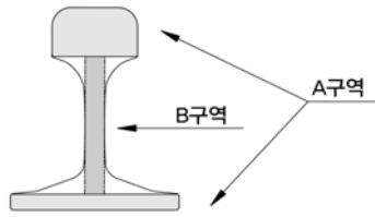
그림 1.3-4 초음파탐상 측정위치
