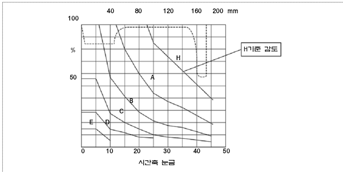
그림 4 거리진폭 특성곡선의 일례
