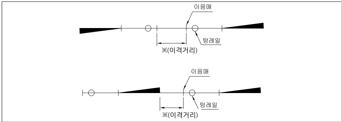
그림 3.3-1 분기기간 이격거리
