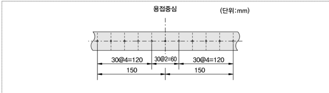
별표 2 경도 측정위치(후열처리 후)
