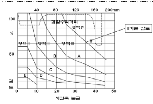
그림 6(a) H기준 감도에 대한 영역구분
