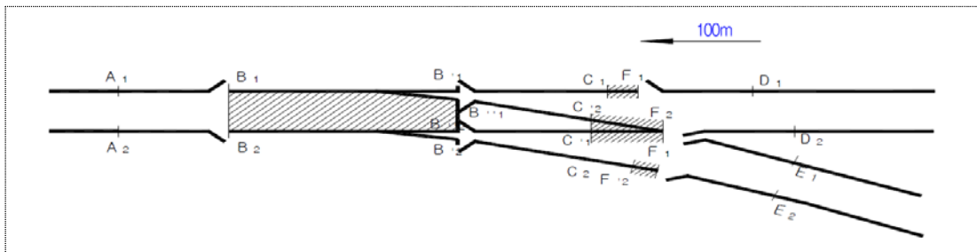
그림 3.3-3 편개 분기기의 장대레일 재설정
