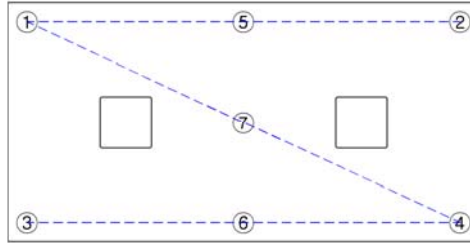
그림 6.3-1 패널 현장반입 시 비틀림 검사 개요도
