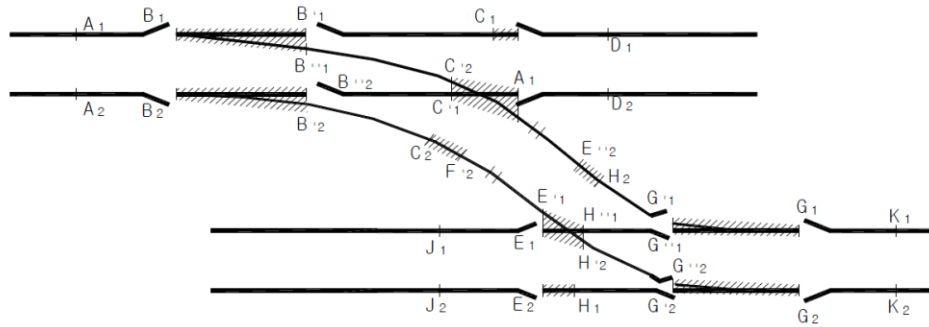
그림 3.3-3 건넘선의 장대레일 재설정
