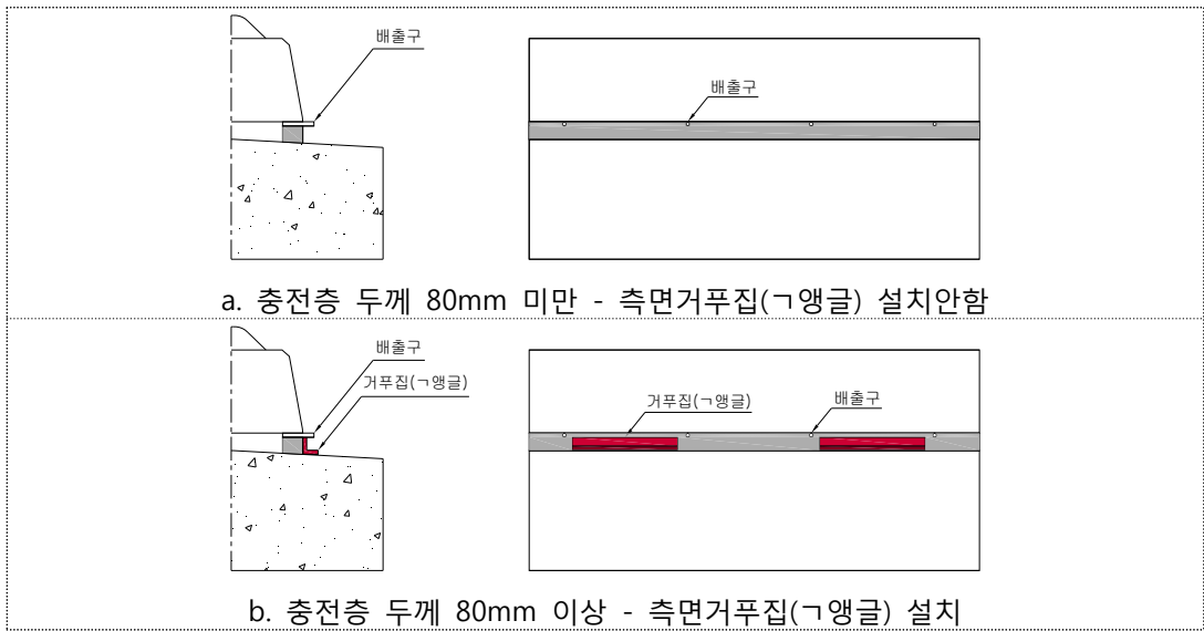
그림 6.3-9 배출구(공기구멍) 위치에 따른 설치방법
