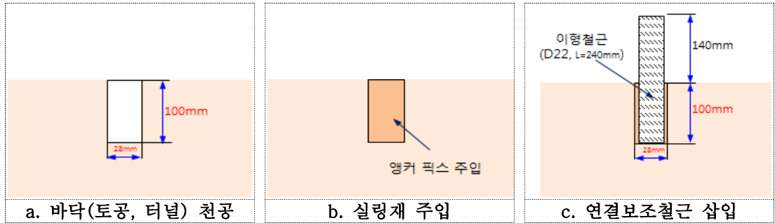
그림 6.3-10 연결보조철근 설치도
