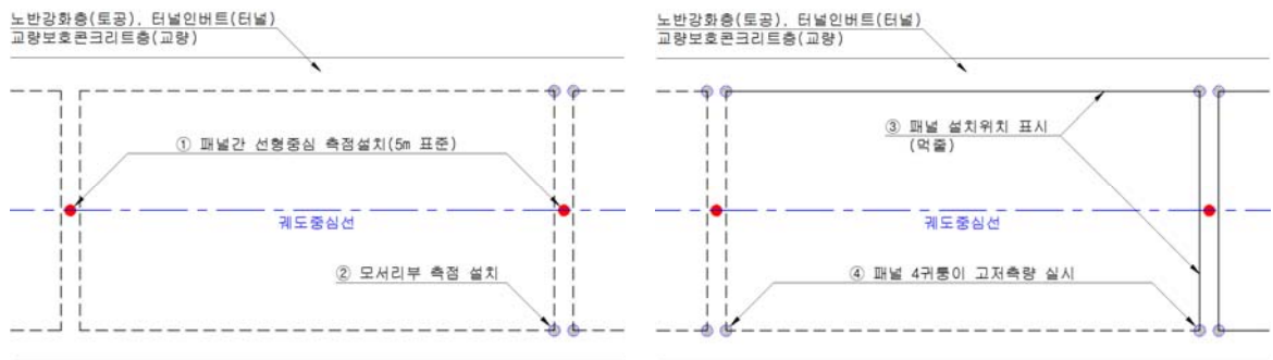
a. 패널 설치용 측량(패널간 중앙부)
