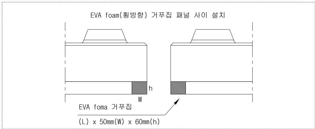
그림 6.3-6 횡방향거푸집 설치 개요도(예시)
