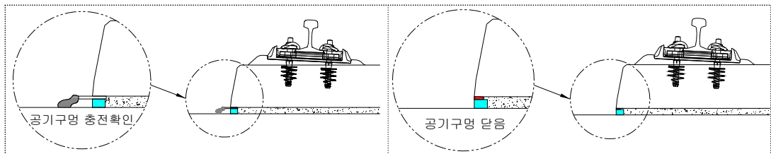
그림 6.3-11 충전재 주입 확인방법
