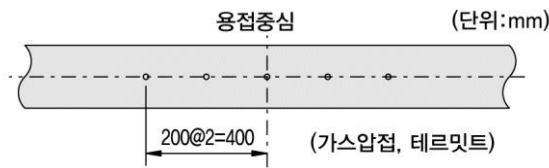
별표 1 경도 측정위치
