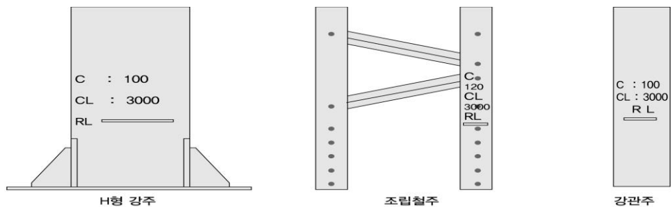
그림 3.3-1 일반철도 전철주 형식별 표기방법(예)
