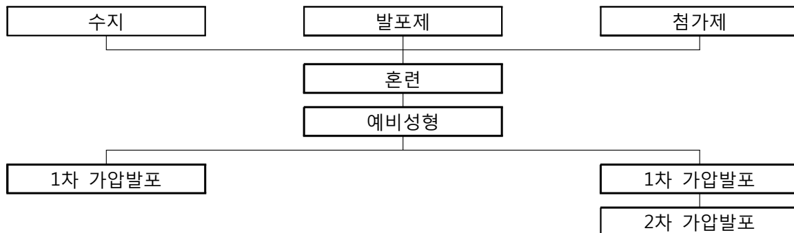
[그림1] EVA foam 제조공정
