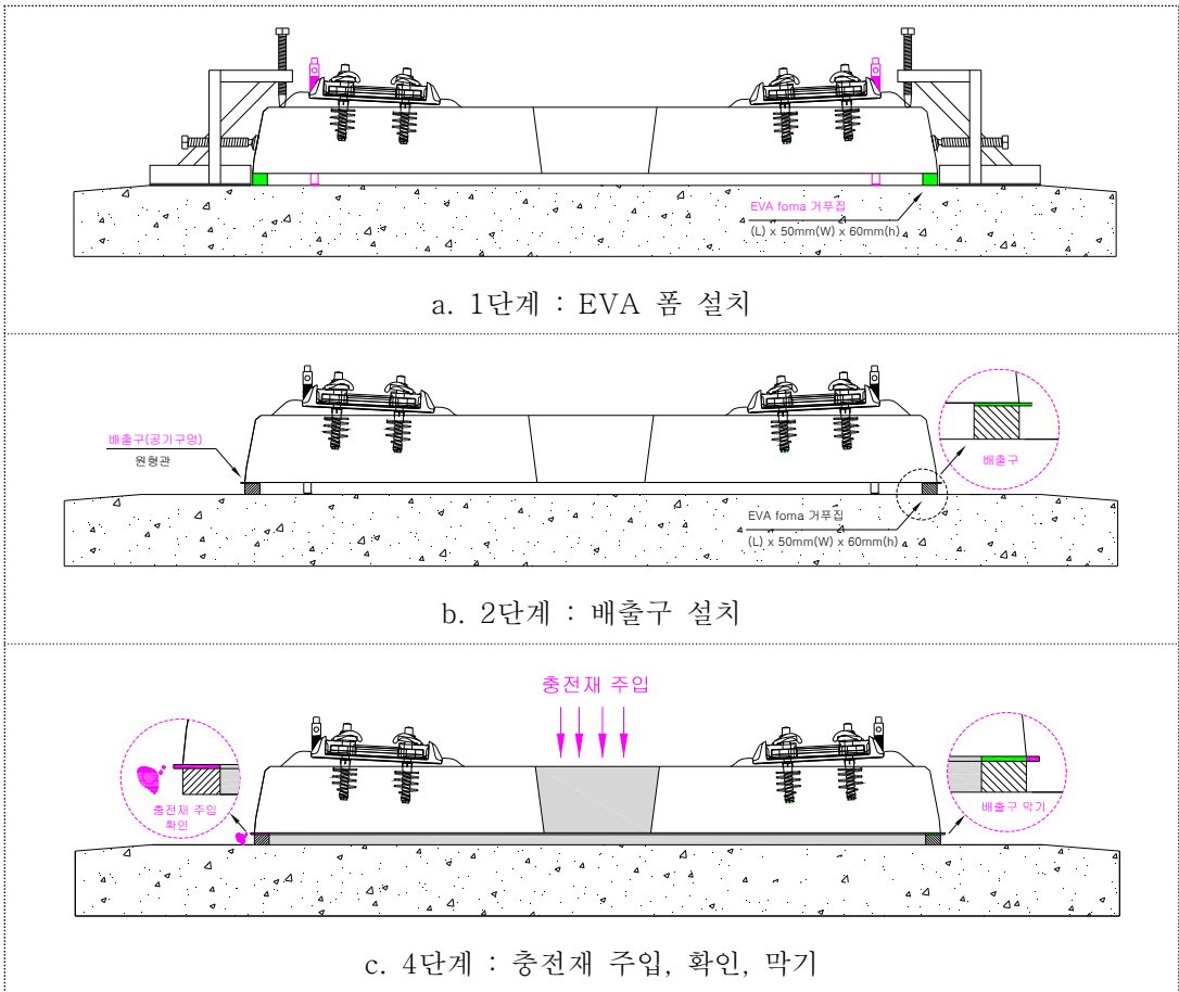
그림 6.3-7 거푸집설치 및 충전재 주입 시공 순서도
