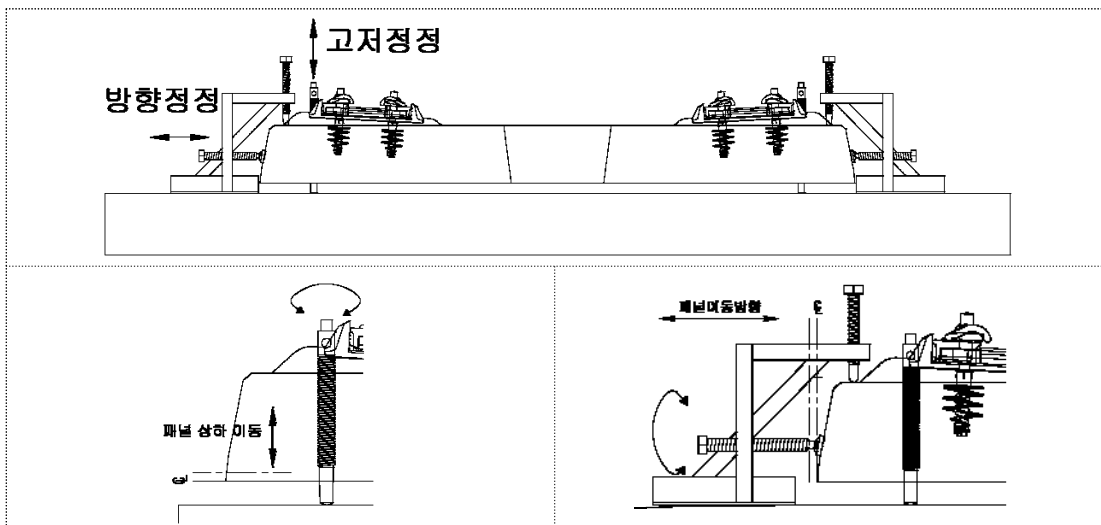
그림 6.3-5 패널 정정(고저, 방향) 상세 개요도
