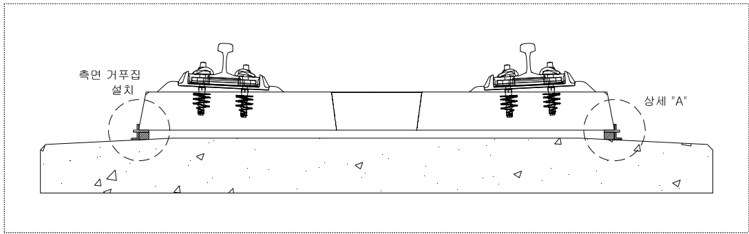
그림 6.3-8 측면(합판) 거푸집 설치 개요도
