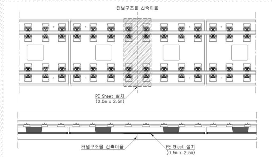
그림 6.3-3 터널 신축이음부 PE Sheet(or Film) 설치 개요도
