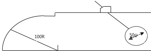
그림 2 굴절각의 측정방법(STB-A1)
