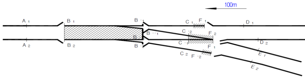
그림 3.3-2 편개 분기기의 장대레일 재설정
